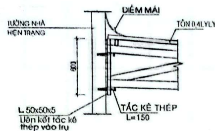
CHI TIẾT LIÊN KẾT ĐẦU KẸO K1 02 VỊ TRÍ; TL 1/25
