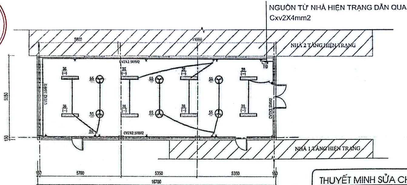
MẶT BẰNG CÁP ĐIỆN TL1/100
