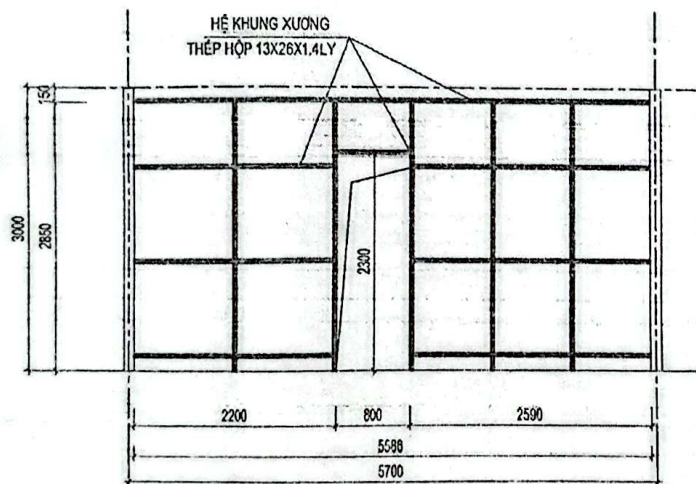
CHI TIẾT KHUNG VÁCH KV2 (CÓ CỬA ĐI Đ2) (02CK) TL1/25
