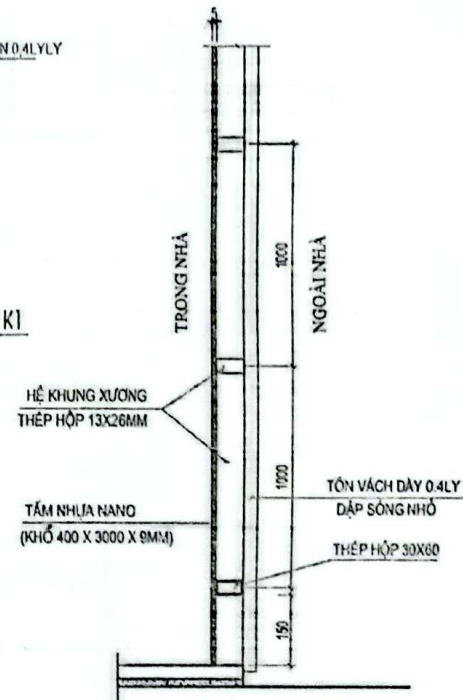
CHI TIẾT ỚP VÁCH; TL 1/5
