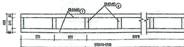
CHI TIẾT GIẢNG K2 TL 1/25 (SI=03CK)
