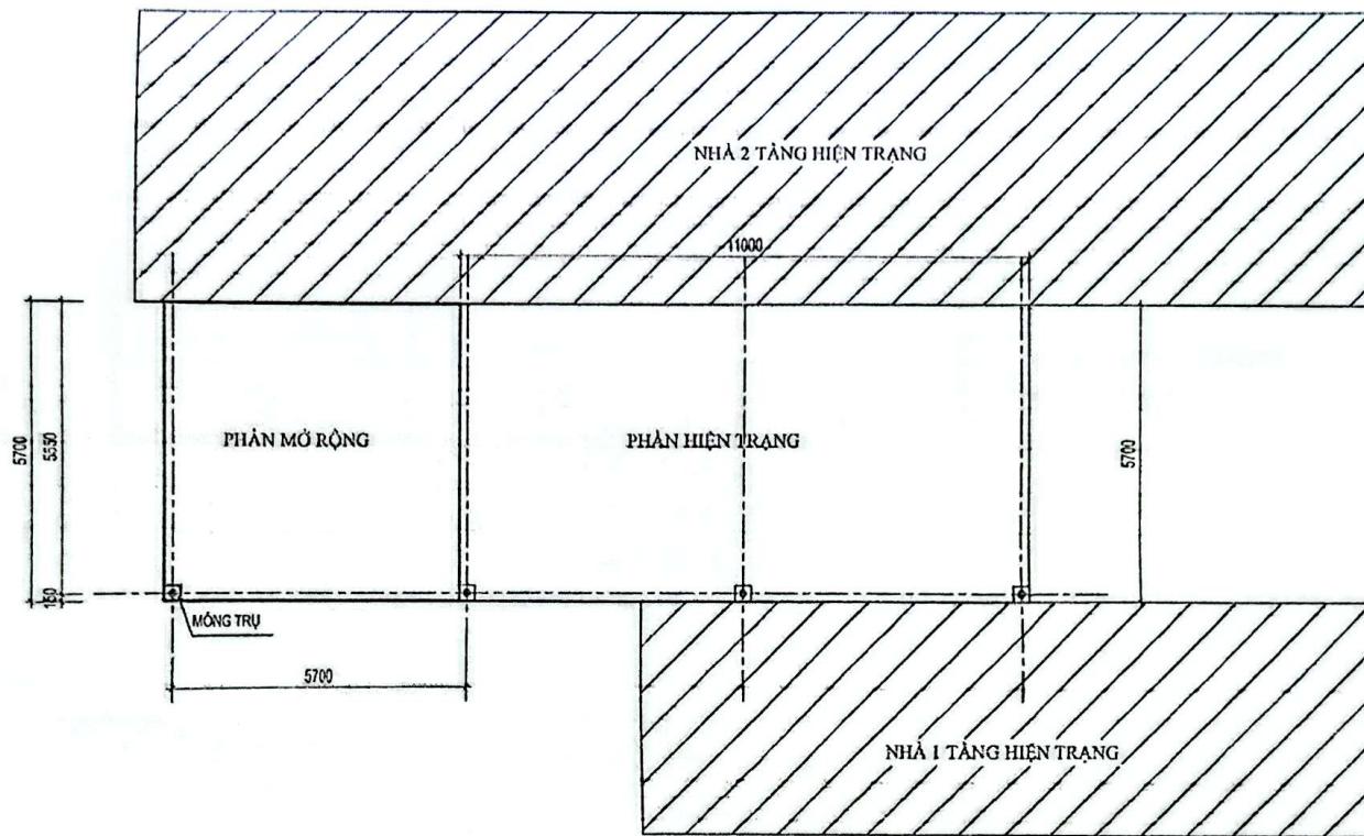
MẶT BẰNG MÓNG CẢI TẠO TL1/100
