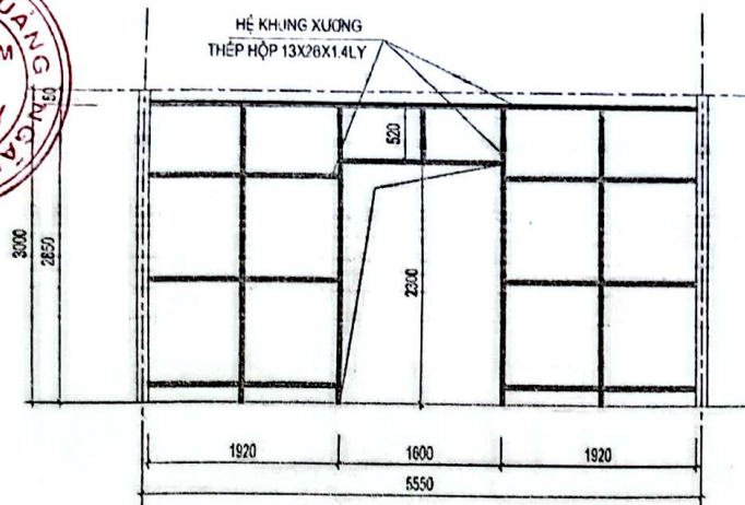
CHI TIẾT KHUNG VÁCH KV1 (CÓ CỬA ĐI Đ1) (01CK) TL1/25
