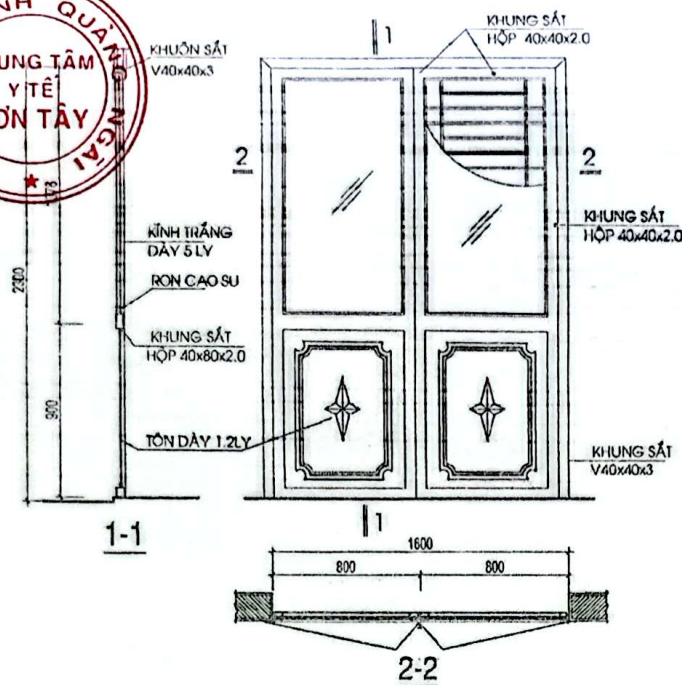
CỬA ĐI Đ1: 01 BỘ
