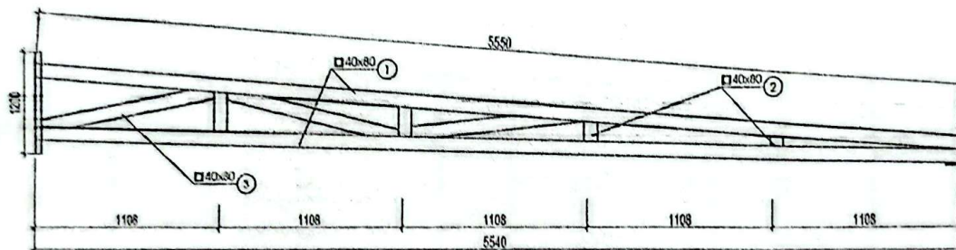
MẶT CẮT A-A; TL 1/50
