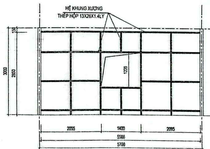
CHI TIẾT KHUNG VÁCH KV2 (CÓ CỬA SỔ S1) (04CK) TL1/25
