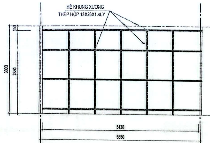
CHI TIẾT KHUNG VÁCH ĐẦU HỒI KV3 (KHÔNG CÓ CỬA) (01CK) TL1/25
