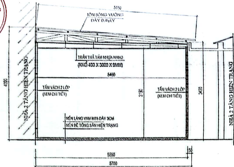
MẶT CẮT A-A; TL 1/50
