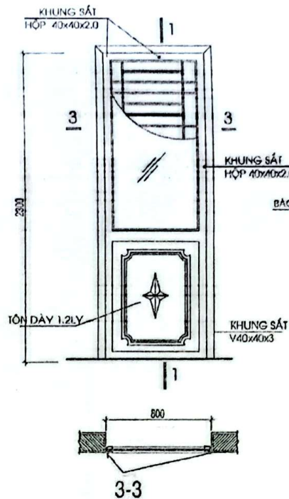
CỬA ĐI Đ2: 02 BỘ
